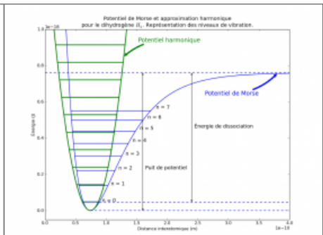
Potentiel de Morse
